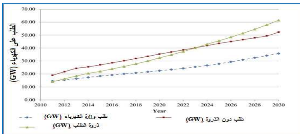
شكل (5) توقعات الطلب على الكهرباء للمدة (2030-2010)
